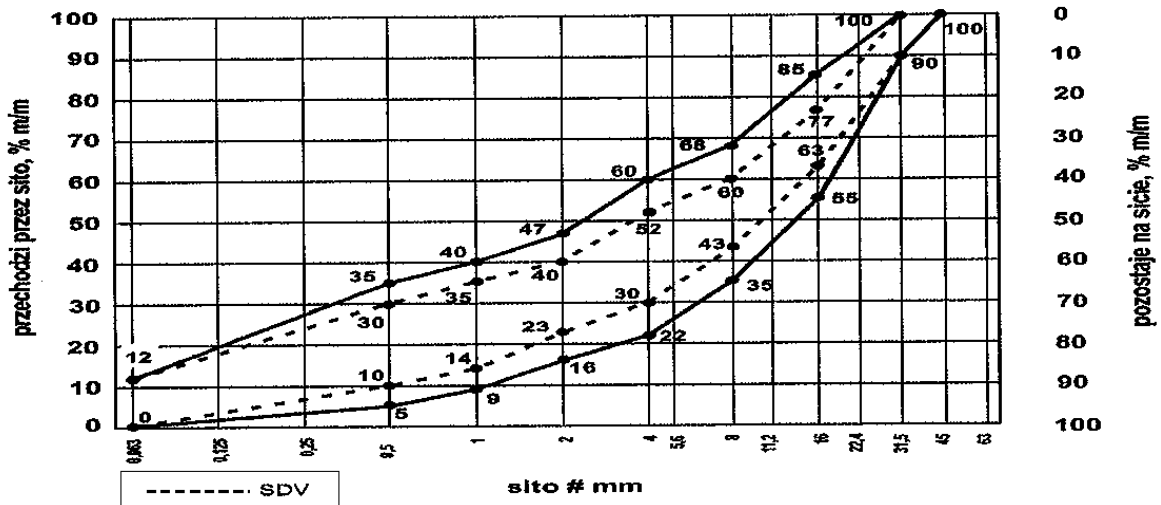
Rysunek 1. Uziarnienie mieszanki niezwiązanej 0/3/1,5 do w-wy podbudowy pomocniczej SDV – obszar uziarnienia, w którym powinna się mieścić krzywa uziarnienia mieszanki (S) deklarowana przez producenta / dostawcę.
